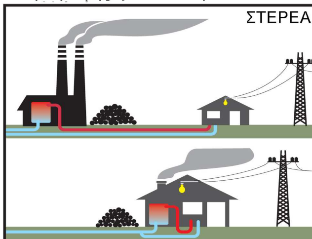
Παραδοσιακό σύστημα παραγωγής ζεστού νερού
